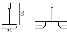
24 LINEAR TEGULAR ribassati di 8/15 mm 8/15 mm lowered
